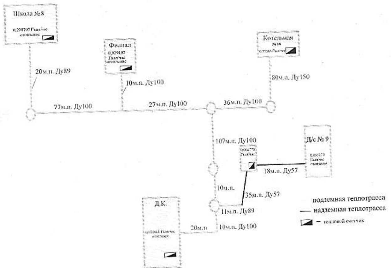
Рисунок 5 Карта котельной в ст. Новопластуновская, ул. Первомайская, 31
